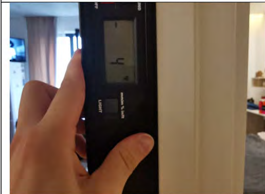
Фото №44. Отклонение коробки деревянного дверного блока в спальне.
