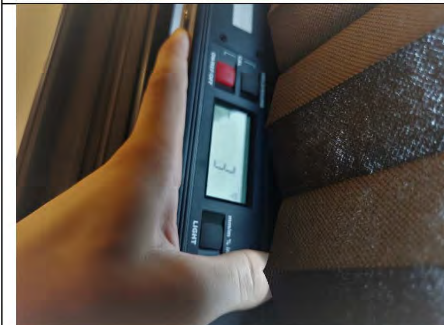
Фото №41. Отклонение металлического оконного блока по уровню вертикальности в спальне.
