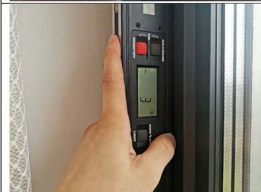
Фото №42. Отклонение металлического оконного блока по уровню вертикальности в кухне.
